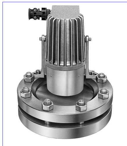
Typ PEL 50 DEH X2 B, 230 V, 50 W, Ex de IIC T4, Ex tD A21 IP65 T130 °C, Ex II 2 G + D, z tarczą zapobiegającą osłepianiu "B", na okrągłym wżerniku wg DIN 28120 DN 150, PN 10, w wersji "Widok i światło przez jeden zespół"
