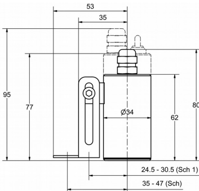
Oprawa oświetleniowa Micro LED TYP MVL R 2 LED E Sch1 , 2W, 24 V AC / DC, z wbudowanym przełącznikiem ON-OFF "E", zamontowany na VETROLUX wzierniku skręcany wg DIN 11851, DN 32, PN 6
