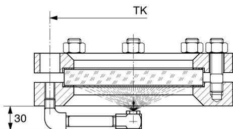
Dysza rozpylająca wybudowana w okrągłym wziernikową DIN 28120.
